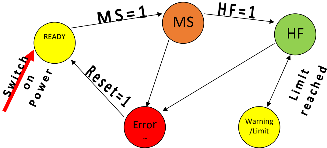
Abbildung 3: Betriebszustände
